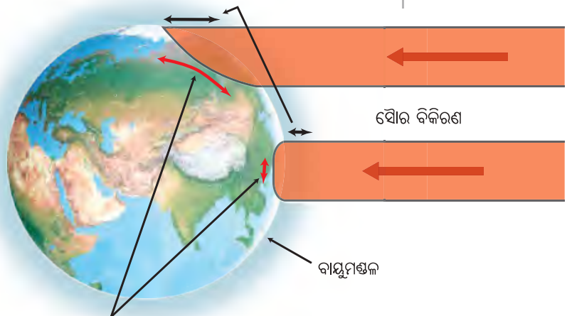
ବାୟୁମଣ୍ଡଳ ବିଷୁବରେଖାଠାରେ ସୌର ରଶ୍ମି କେନ୍ଦ୍ରିତ ହୋଇଥାଏ । କିନ୍ତୁ ମେରୁ ନିକଟରେ ବିଷୁବିତ ଅଞ୍ଚଳର ବିଚ୍ଛିନ୍ନ ହୋଇଥାଏ ।
