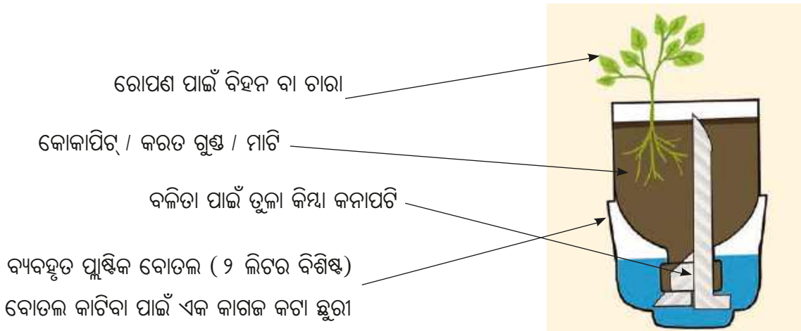
ଚିତ୍ର ୧.୩ (ଖ) ଅବଶୋଷଣ ପ୍ରଣାଳୀ ଆଧାରିତ ହାଇଡ୍ରୋପୋନିକ୍ସ ବ୍ୟବସ୍ଥା
