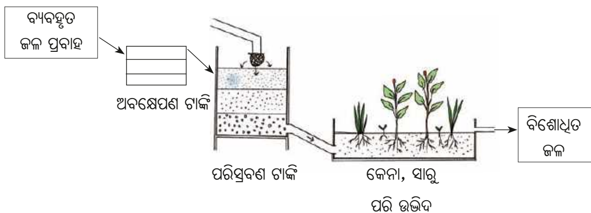
ଚିତ୍ର ୫.୧୬ : ଅପଚୟ ଜଳର ପୁନଃ ବ୍ୟବହାର ପାଇଁ ପ୍ରାକୃତିକ ଜଳ ଅବଶେଷ ପ୍ରଣାଳୀ
